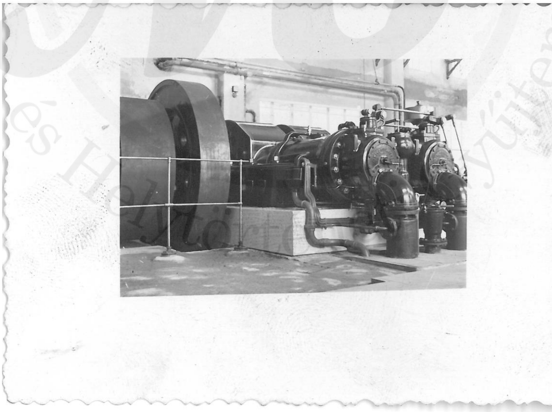
11. számú melléklet: Forgórostélyos barnaszén generátor
